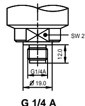
G 1/4 A
