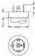
ISO 4400 (IP 65)
